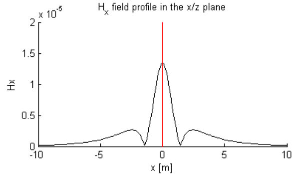
Fig. 8 horizontal dipole
